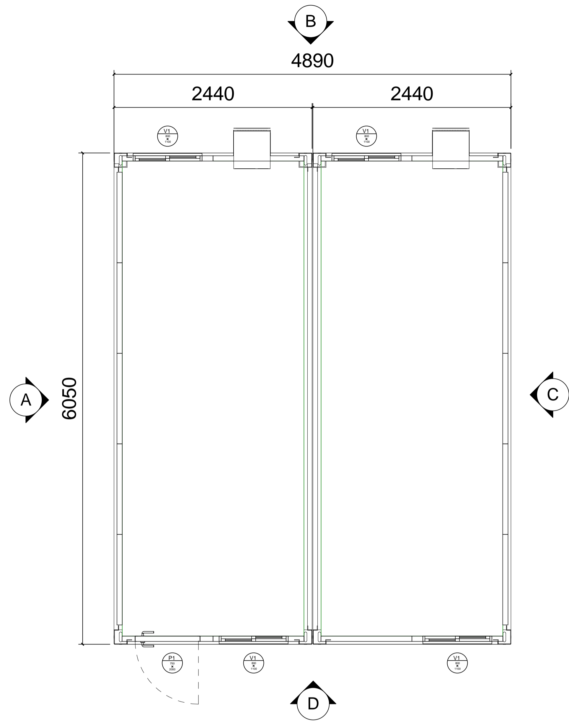
PLANTA DE ARQUITECTURA Esc.: 1:25
