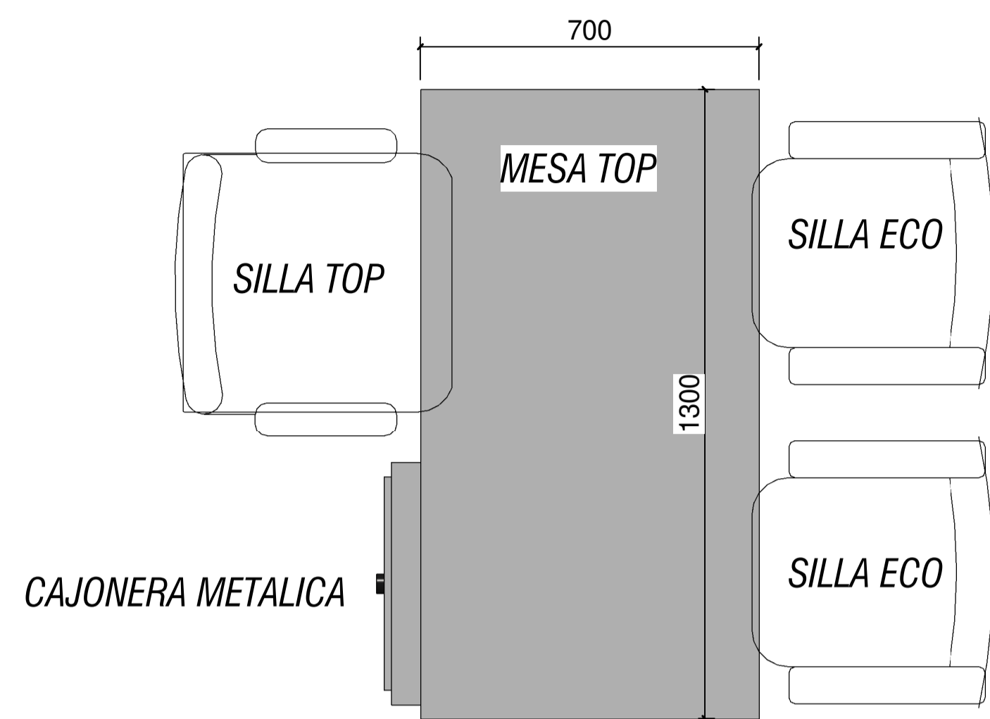
PLANTA DE ARQUITECTURA Esc.: 1:10 COMBO OFICINA DOBLE
