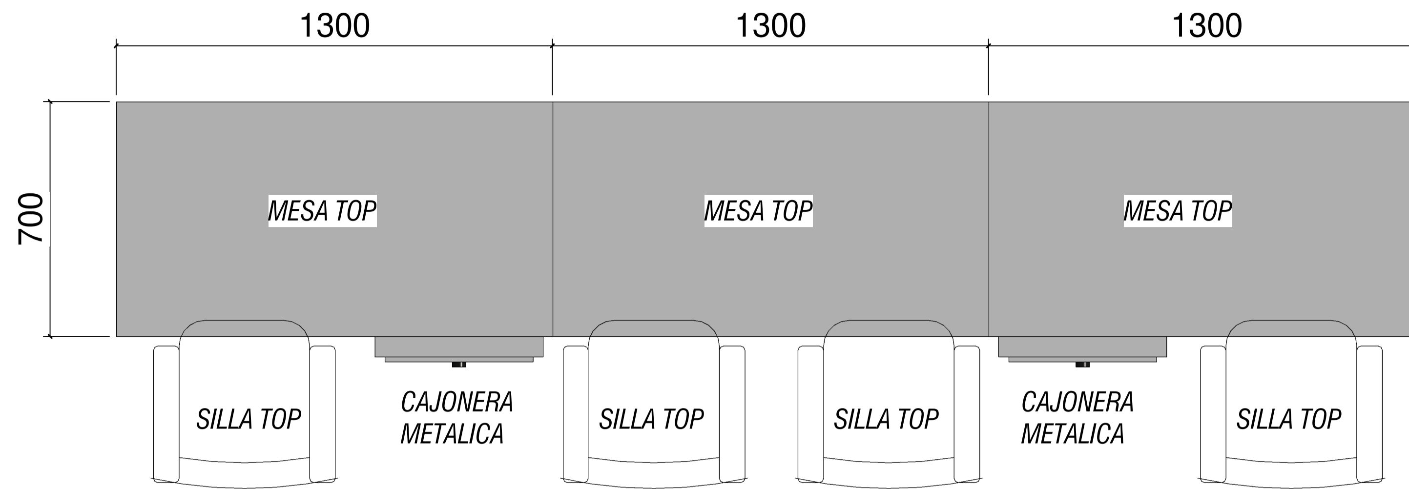
PLANTA DE ARQUITECTURA Ebc.: 1:10 COMBO OFICINA PERIMETRAL TOP
