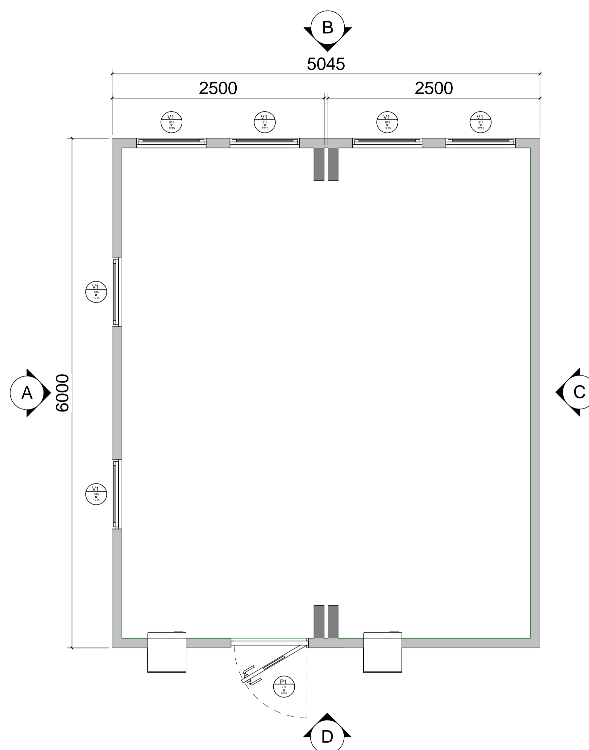
PLANTA DE ARQUITECTURA Esc.: 1:25 MODULOS 30m 2
